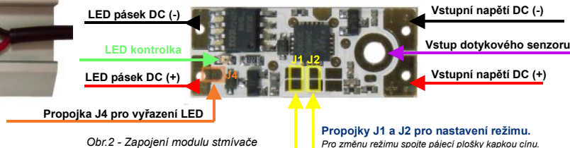
Obr. 2 - Zapojení modulu stmívače
